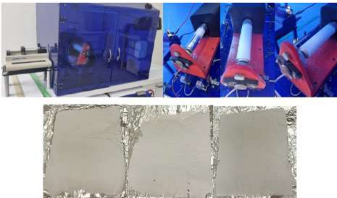
Figura 1 Proceso de electrohilado
