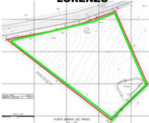
PLANTA GENERAL DEL PERÍMETRO Escala: 1:500
