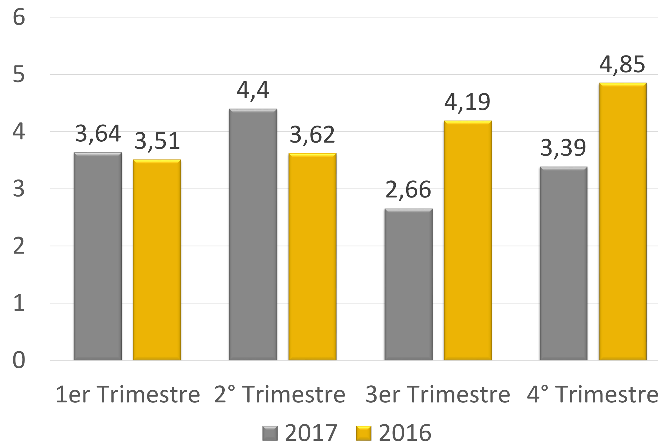
Consumo kW/h por m 2 construido
